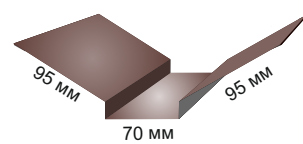
Накладка ендовы
