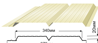
С ЦЕНТРАЛЬНОЙ ПЕРФОРАЦИЕЙ
