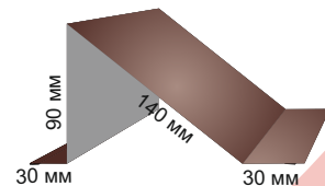
Снегозадержатель
