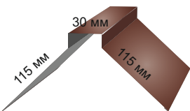
Конек фигурный
