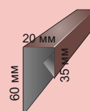
Наличник сложный
