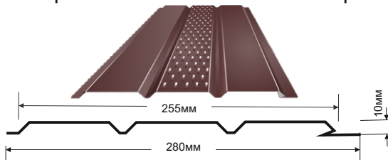
С ЦЕНТРАЛЬНОЙ ПЕРФОРАЦИЕЙ
