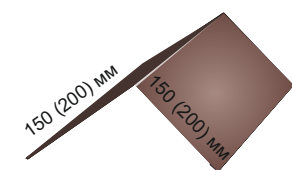
Конек плоский
